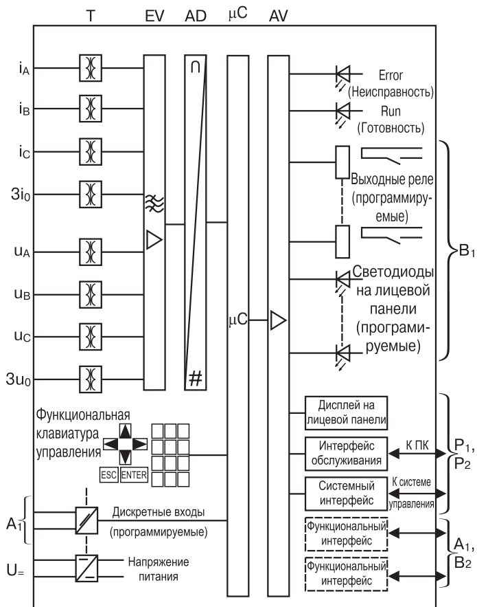
Рис. 2. Структурная схема устройства 7SD6 по [10]
