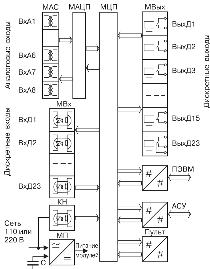
Рис. 1. Структурная схема устройств серии БМРЗ
